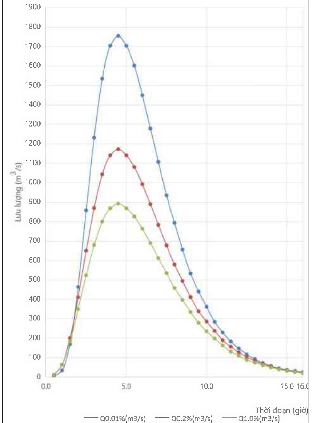
Hình PL.2.2 : Hình vẽ quá trình lũ đến hồ Suối Trầu ĐƯỜNG QUÁ TRÌNH LŨ ĐẾN HỒ SUỐI TRẦU
