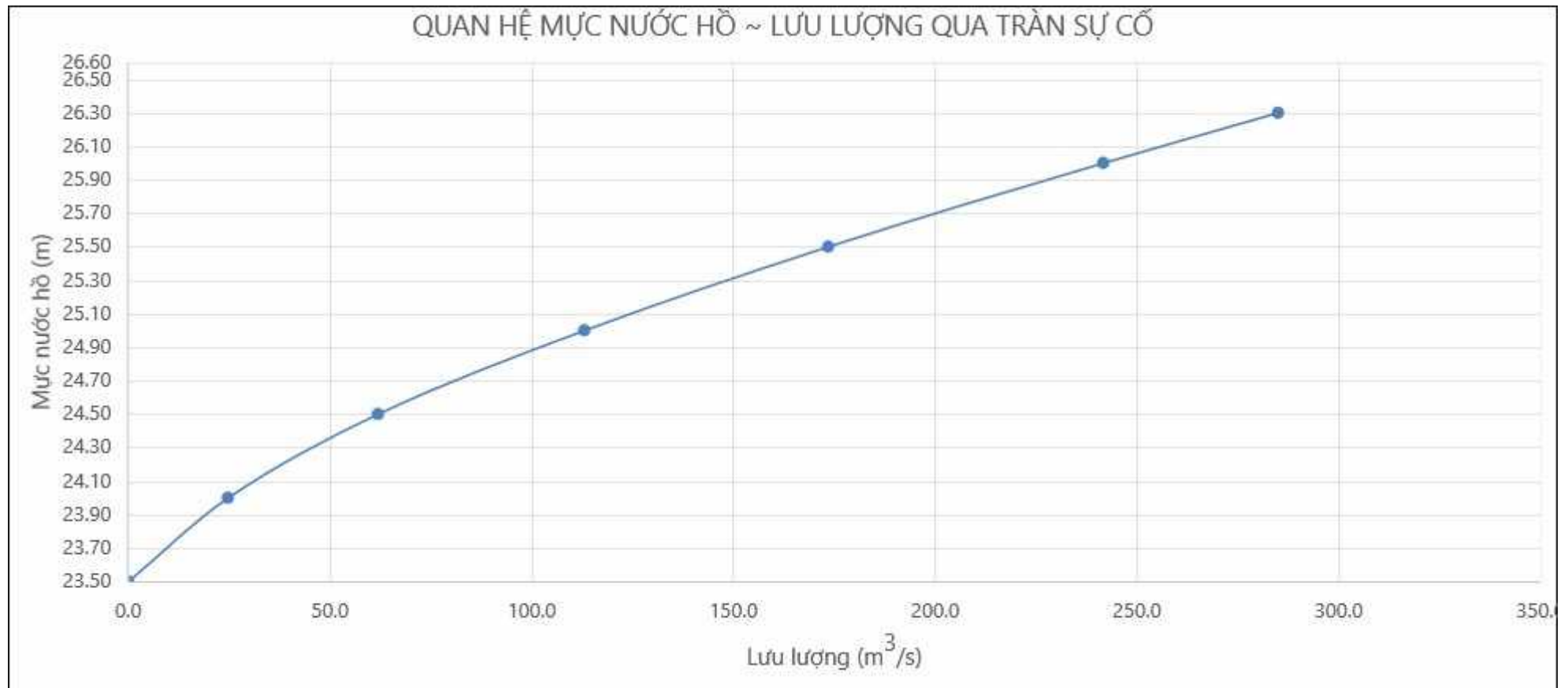
Hình PL 5.5: Lưu lượng qua tràn ~ Mực nước hồ (Tràn sự cố)
