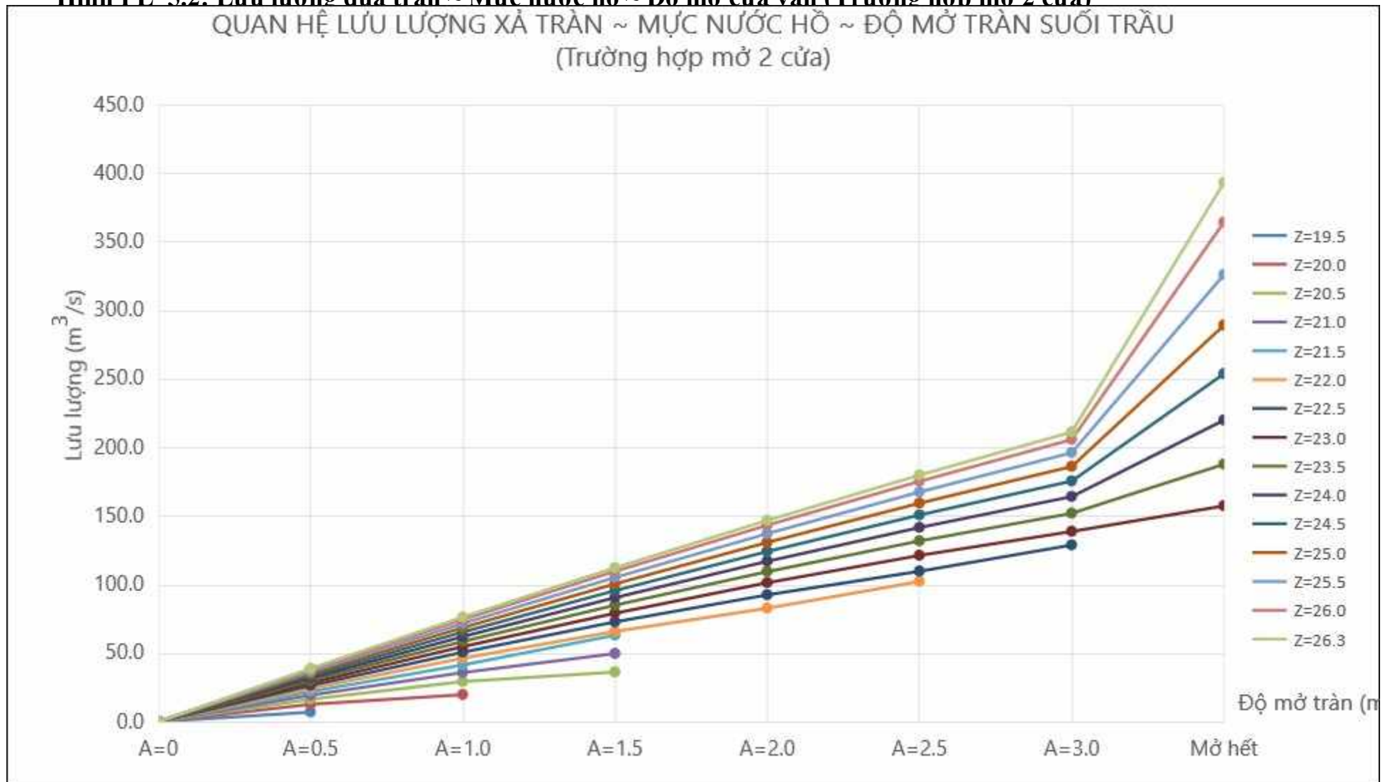
Hình PL 5.2: Lưu lượng qua tràn ~ Mức nước hồ ~ Độ mở cửa van (Trường hợp mở 2 cửa)
