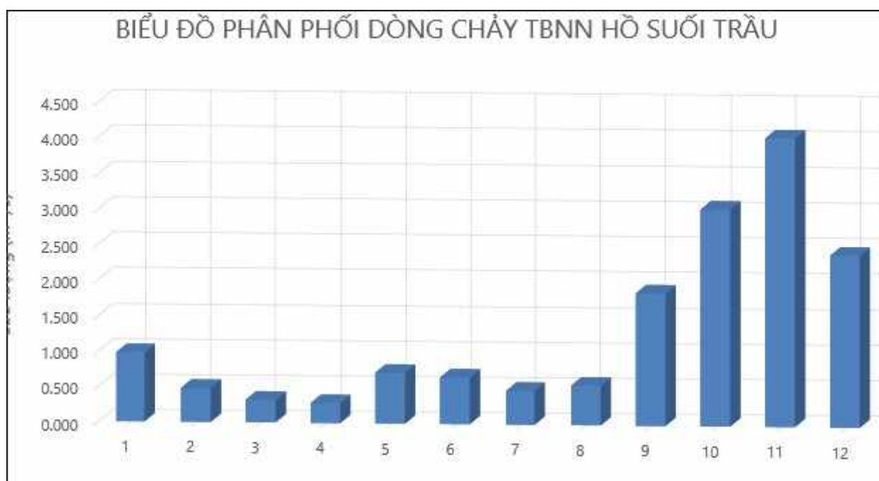
Hình PL 2.1 : Hình vẽ biểu đồ dòng chảy TBNN đến hồ Suối Trầu
