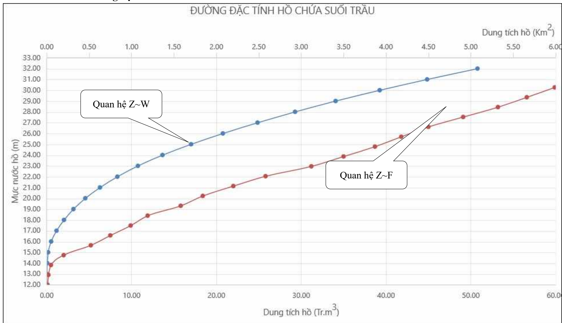
Hình PL8.1 Đường đặc tính hồ chứa nước Suối Trầu
