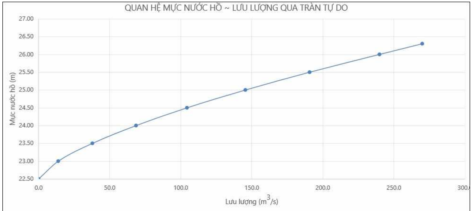
Hình PL 5.4: Lưu lượng qua tràn ~ Mực nước hồ (Tràn tự do)
