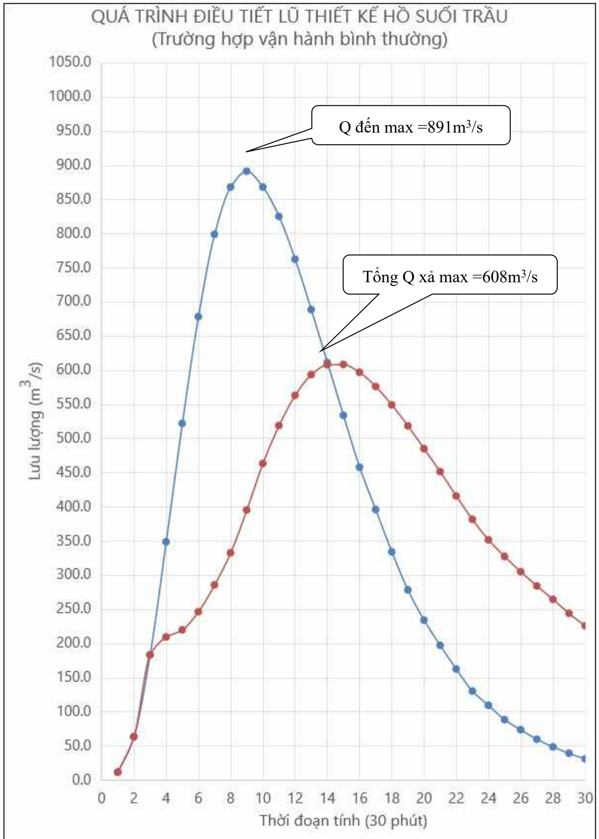
Hình PL 4.1: Quá trình điều tiết lũ thiết kế hồ suối Trầu (Trường hợp vận hành bình thường)
