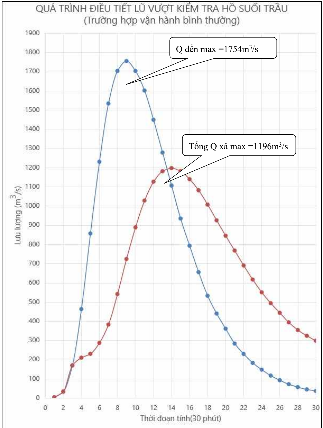
Hình PL 4.5: Quá trình điều tiết lũ vượt kiểm tra
