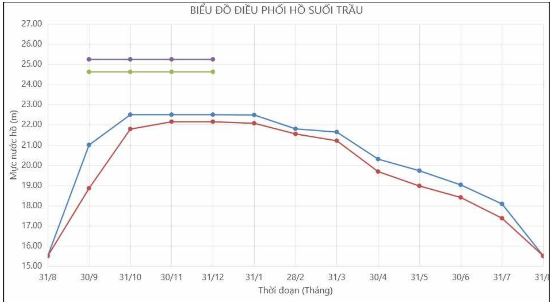
Hình PL7.1 Biểu đồ điều phối hồ chứa nước Suối Trầu
